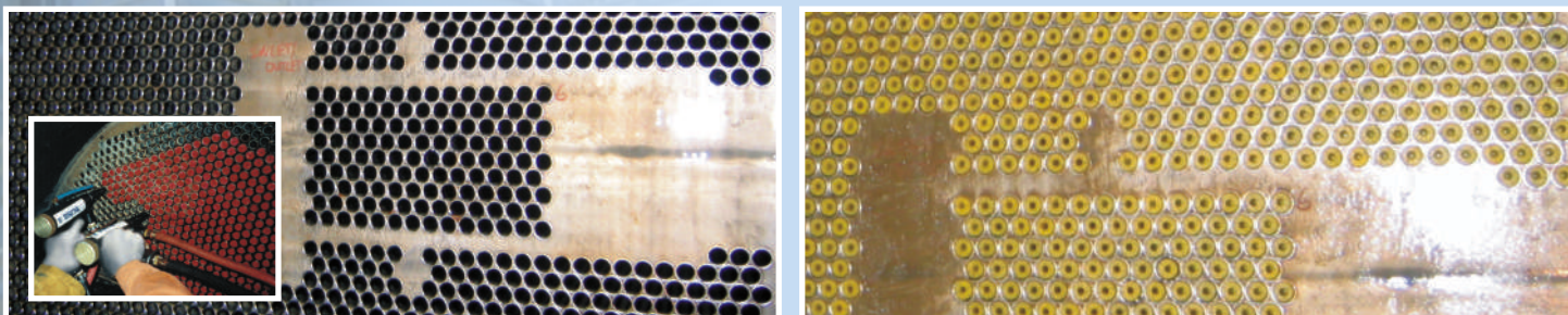
Limpeza através do disparo de esfregadores por pistola
